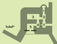
Bunkier typu Regelbau 514 – Pohulanka
